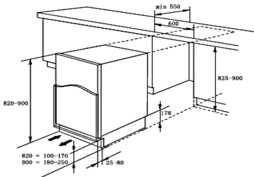
Abbildung 1 - Einbaumaße
