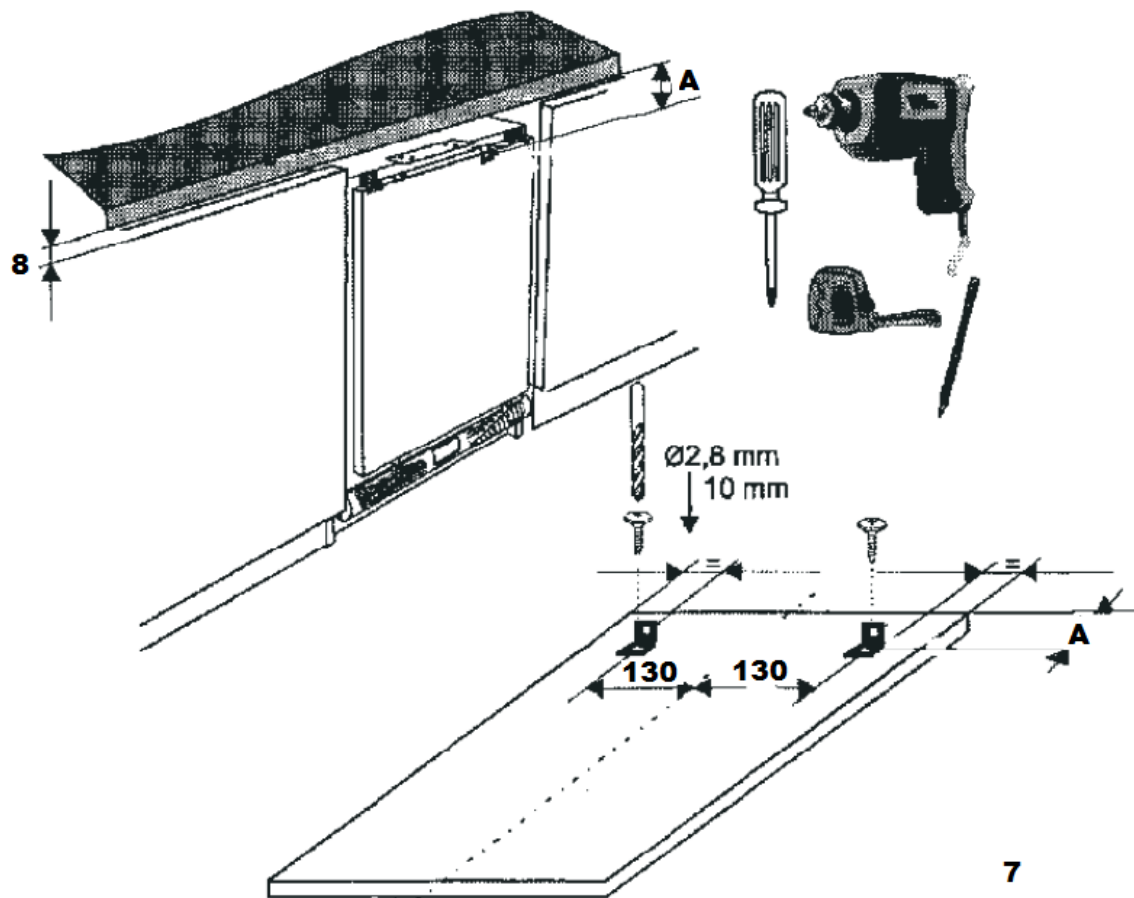
Abbildung 7/8 Befestigung der Tür des Einbaumöbels
