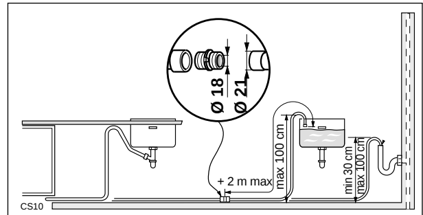
Führung des Ablaufschlauches mit Ablaufbelüftung bei hocheingebauten Geschirrspülern
