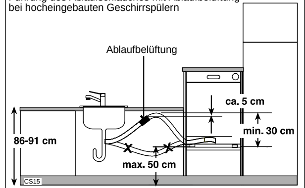
Führung des Ablaufschlauches mit Ablaufbelüftung bei hocheingebauten Geschirrspülern
